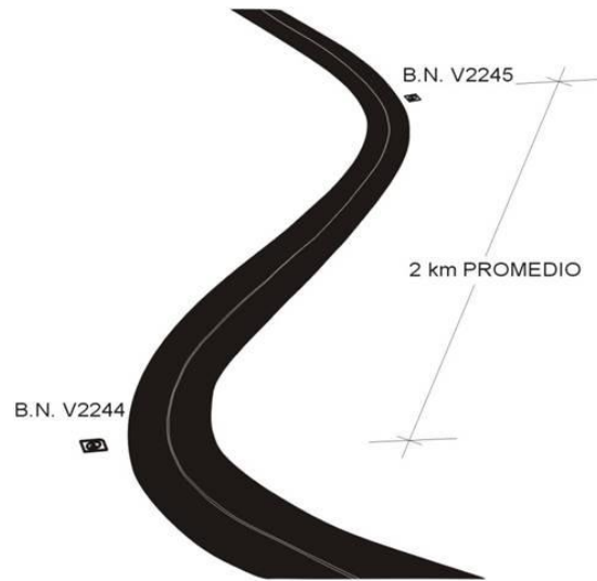
Figura 2. Ubicación de Bancos de Nivel sobre vías de comunicación con curvas horizontales
