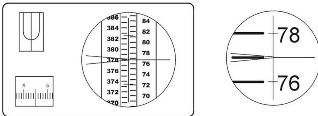
Figura 27. Imagen de ejemplo de los elementos de una Nivelación Simple
